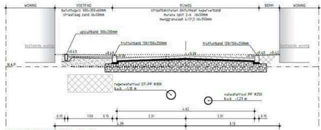
DWARSPROFIEL C-C SCHAAL 1:50
